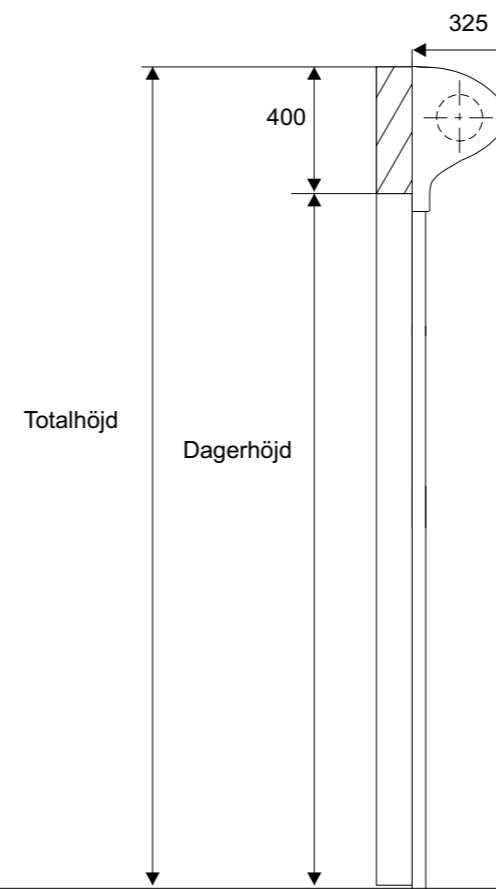
Sektion A-A
